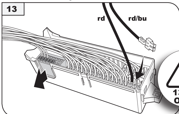
E-Satz rd/bu +30 → freie Kammer e-kit rd/bu +30 → free fuseslot
