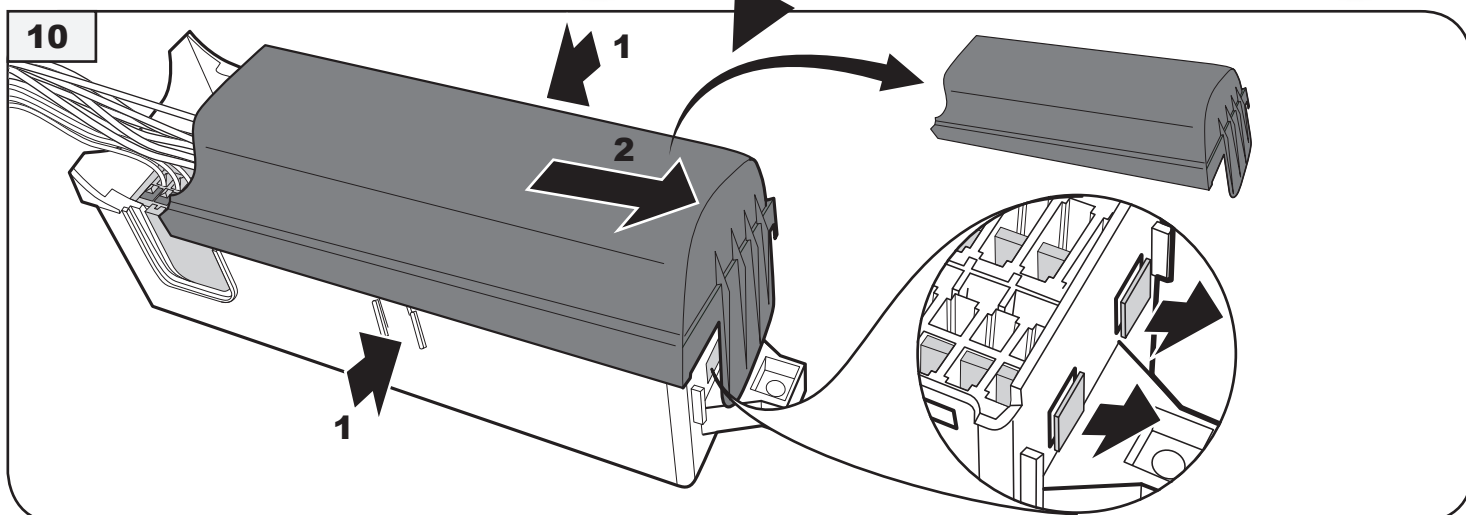
Sicherungskasten fusebox
