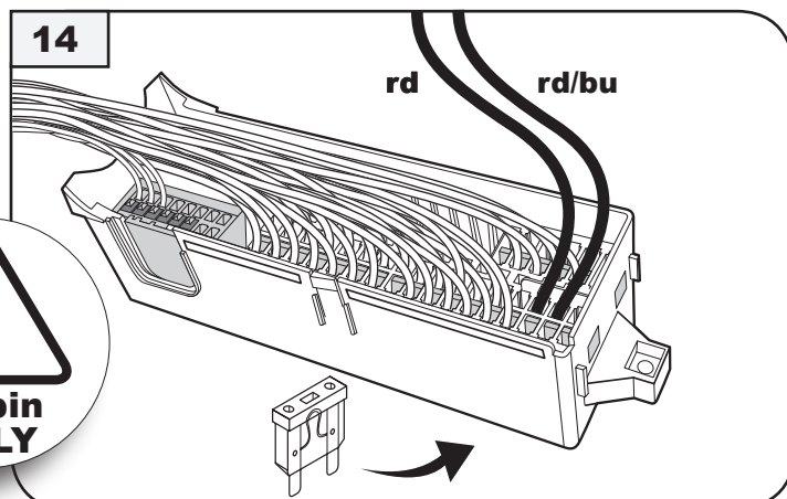
Sicherung 20A fuse 20A
