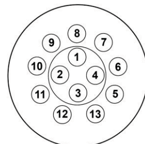
Подключение проводов в 13-полюсной розетке
