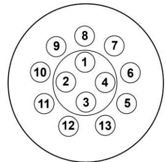
Johtojen liittäminen 13-napaiseen pistorasiaan
