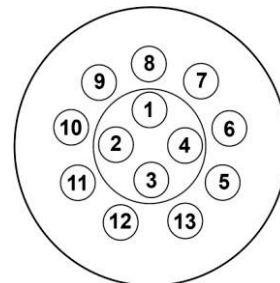
Laidų pajungimas 13 – pavažų lizdas
