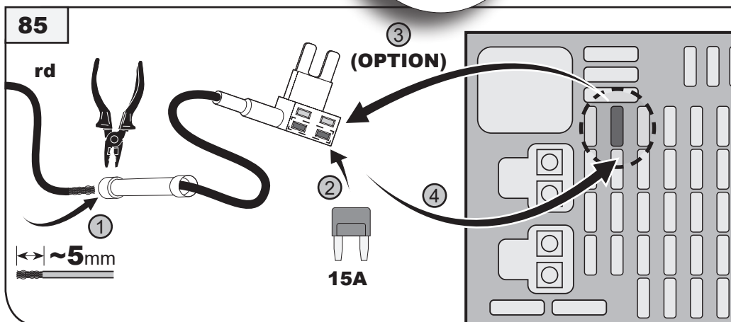
Sicherung 15A → E-Satz rd → Kammer fuse 15A → e-kit rd → fuseslot
