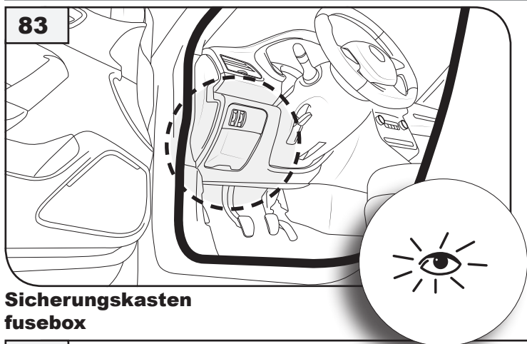
Sicherung 15A → E-Satz rd → Kammer 10 fuse 15A → e-kit rd → fuseslot 10
