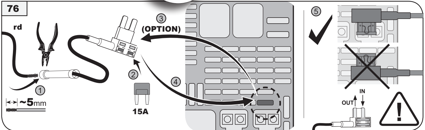
Sicherung 15A → E-Satz rd → Sicherungskasten fuse 15A → e-kit rd → fusebox
