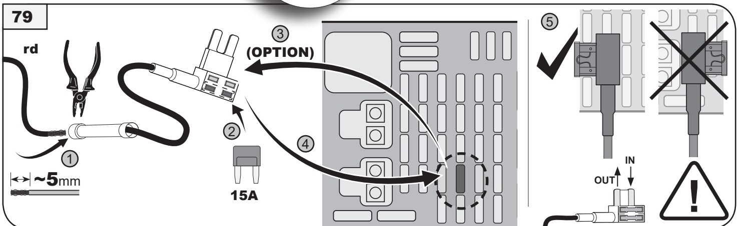
Sicherung 15A → E-Satz rd → Kammer 10 fuse 15A → e-kit rd → fuseslot 10
