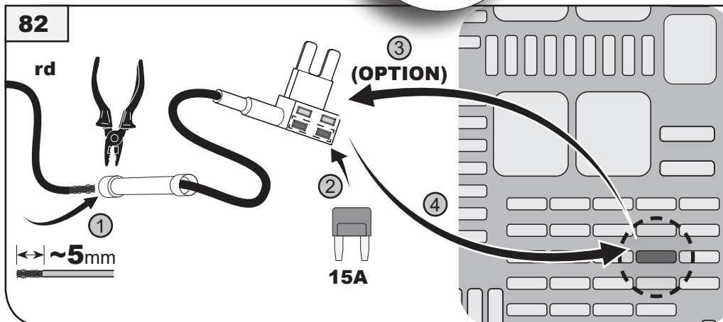
Sicherung 15A → E-Satz rd → Kammer 10 fuse 15A → e-kit rd → fuseslot 10
