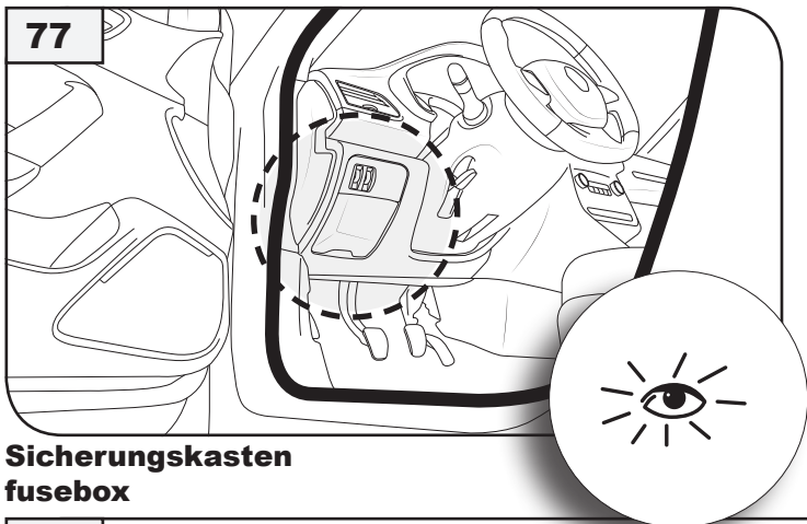
Sicherung 15A → E-Satz rd → Sicherungskasten fuse 15A → e-kit rd → fusebox
