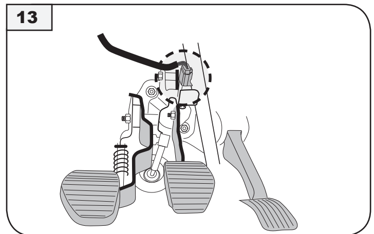
Brems Stecker brake switch
